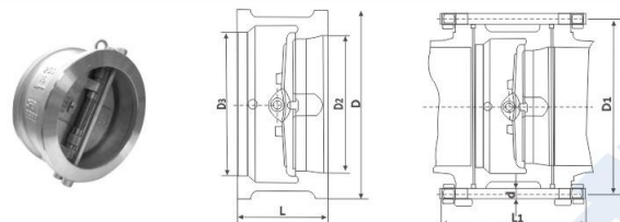
PN10 H76型对夹式不锈钢止回阀
