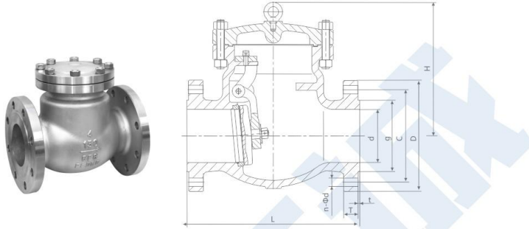
主要尺寸 Dimensions of Flanged end
